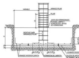
ZAPATA AISLADA
